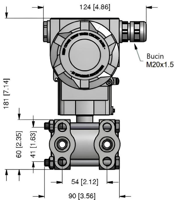
DPT 200 SEM DISPLAY
