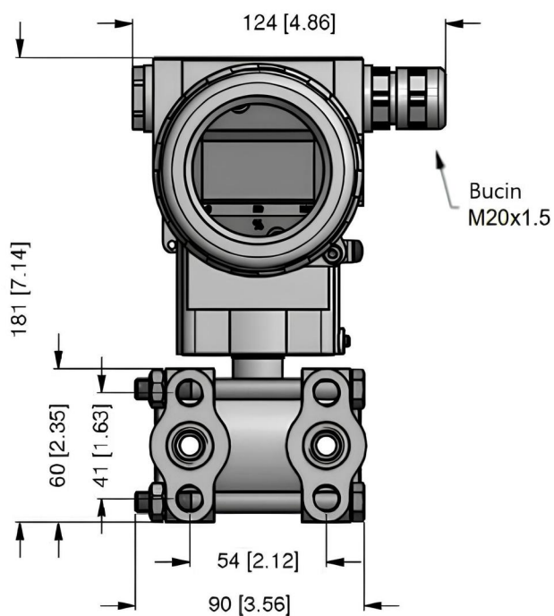
DPT 200 COM DISPLAY
